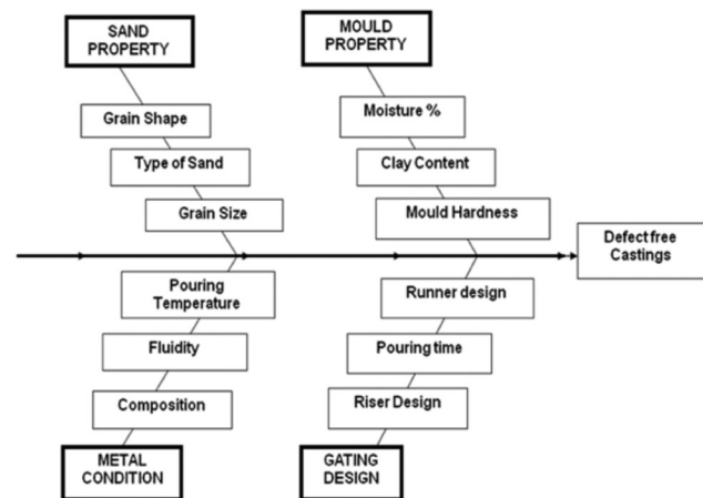
Figura 2. Diagrama Ishikawa para el análisis de los defectos en piezas fundidas.
