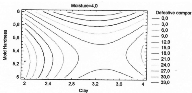
Figura 5. Gráfico de Contornos de la Superficie de Respuesta Estimada.
