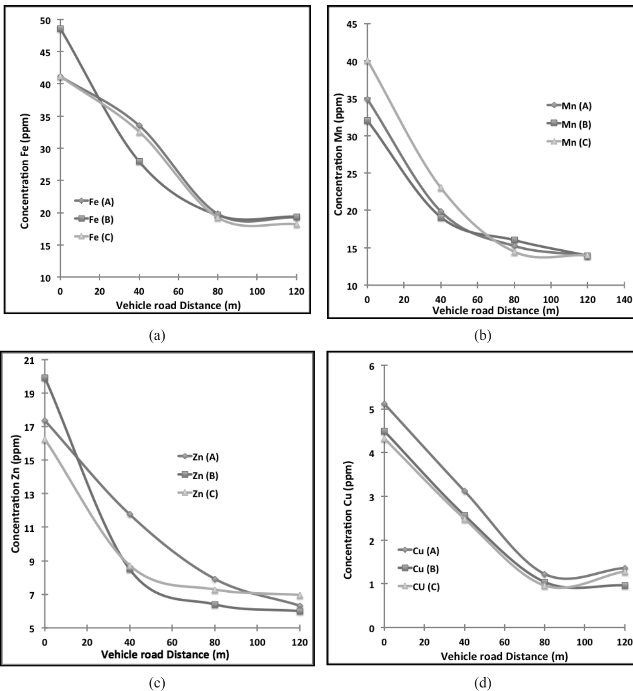
Figura 2. Contenido de cada muestra dependiendo de su ubicación de muestreo de la figura 1: (a) Fe, (b) Mn, (c) Zn y (d) Cu.
